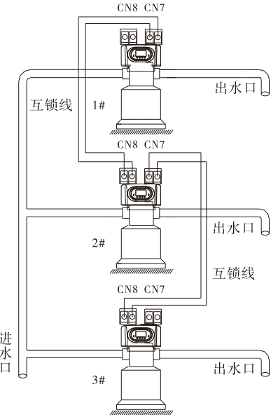
图3-12 同时供水，分别再生
