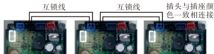
图3-9 互锁的接线图
