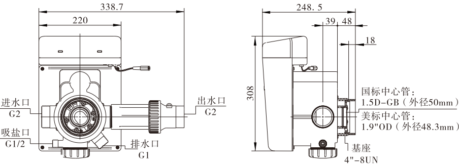
65610结构图
