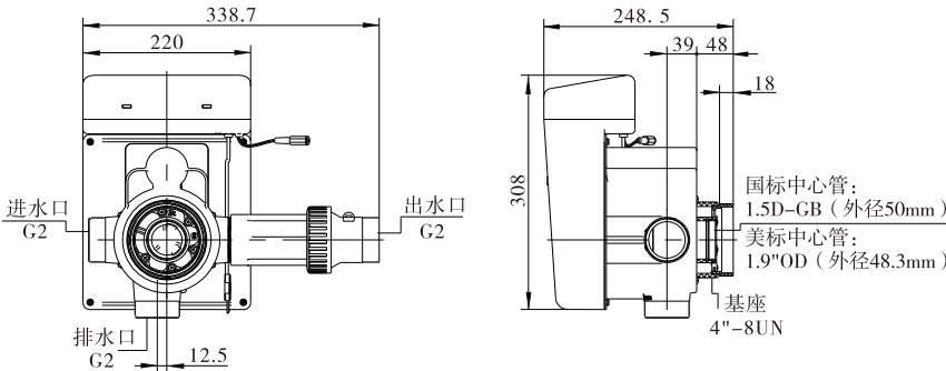
55610结构图
