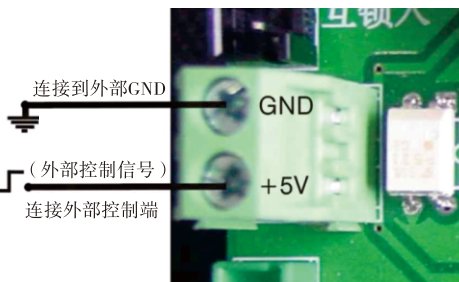
3-11 远程控制端口的接线图
