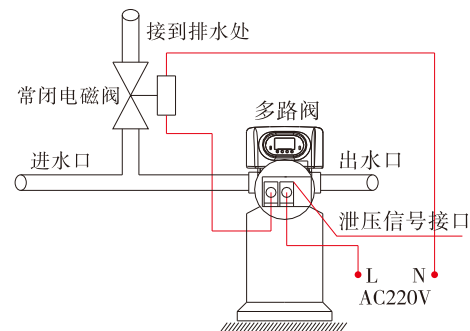
图3-10 泄压端口的接线图
