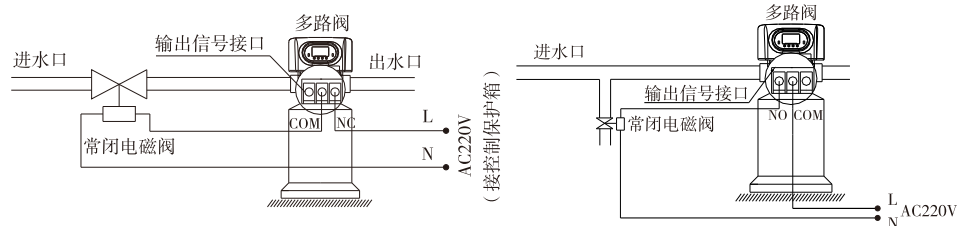
图3-2 控制进口电磁阀的接线图
